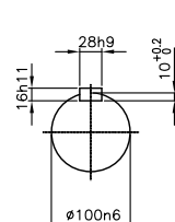
INPUT SHAFT
