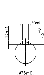
INPUT SHAFT
